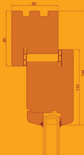
przekrój skrzydła i ościeżnicy DZK 2007 TO
