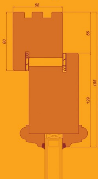
przekrój skrzydła i ościeżnicy DZK 2007
