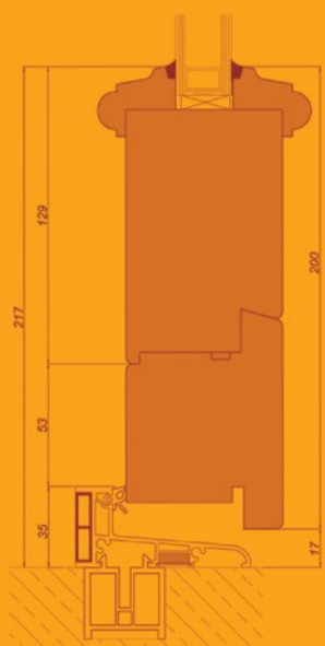
przekrój skrzydła i ościeżnicy DZK 2007
