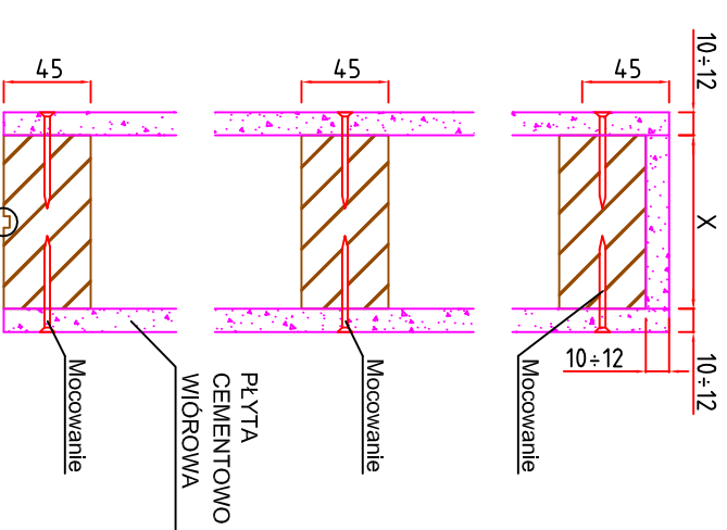
A-A
